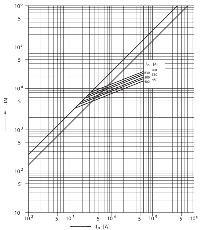
Omezovací charakteristika P50U10, P50V10 aR
